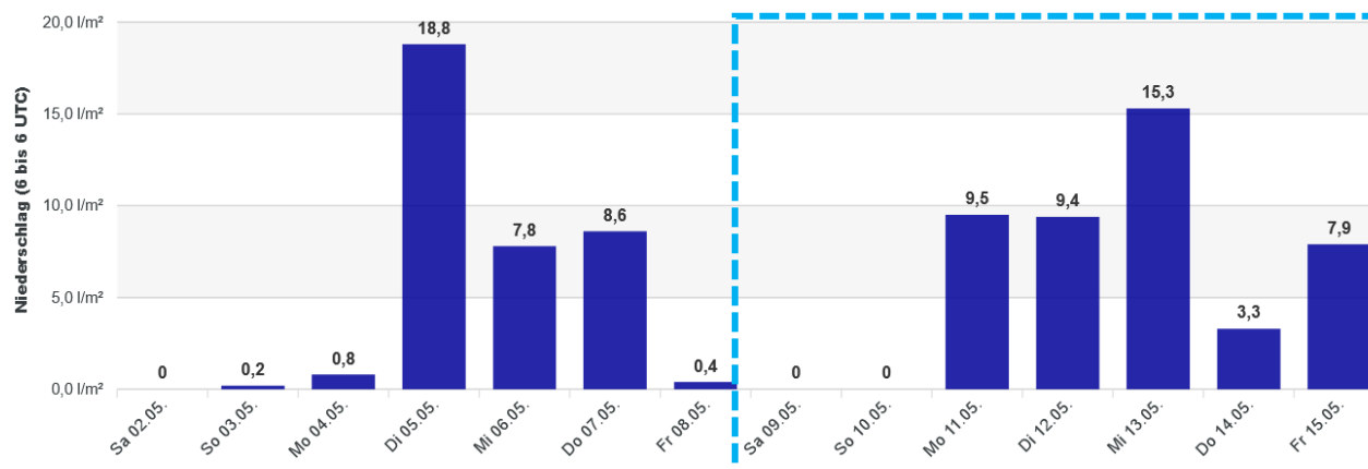
Abb. 3: Übersicht zum Niederschlag an der Wetterstation Suhl-Gehlborg – 14-Tage-Rückblick einschließlich Aktionszeitraum Loungemöbel 09.–15.05.2026; © Wetterkontor, Datenquelle DWD; Quelle: https://www.wetterkontor.de , Abruf 20.05.2026
